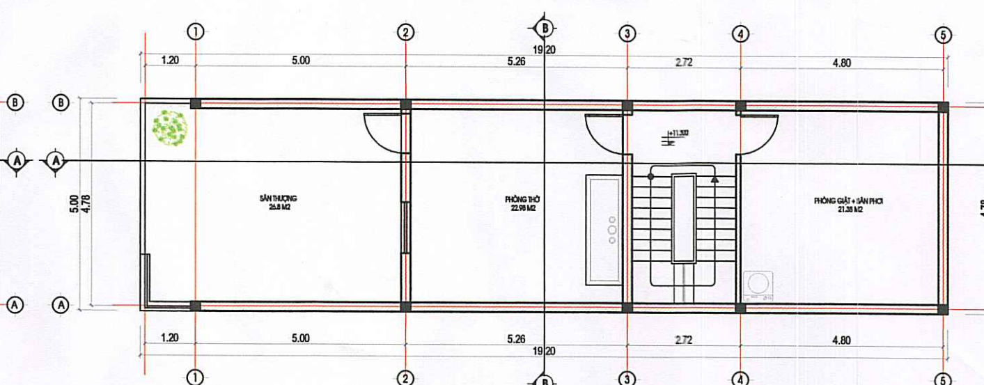
MẶT BẰNG TẦNG 4
