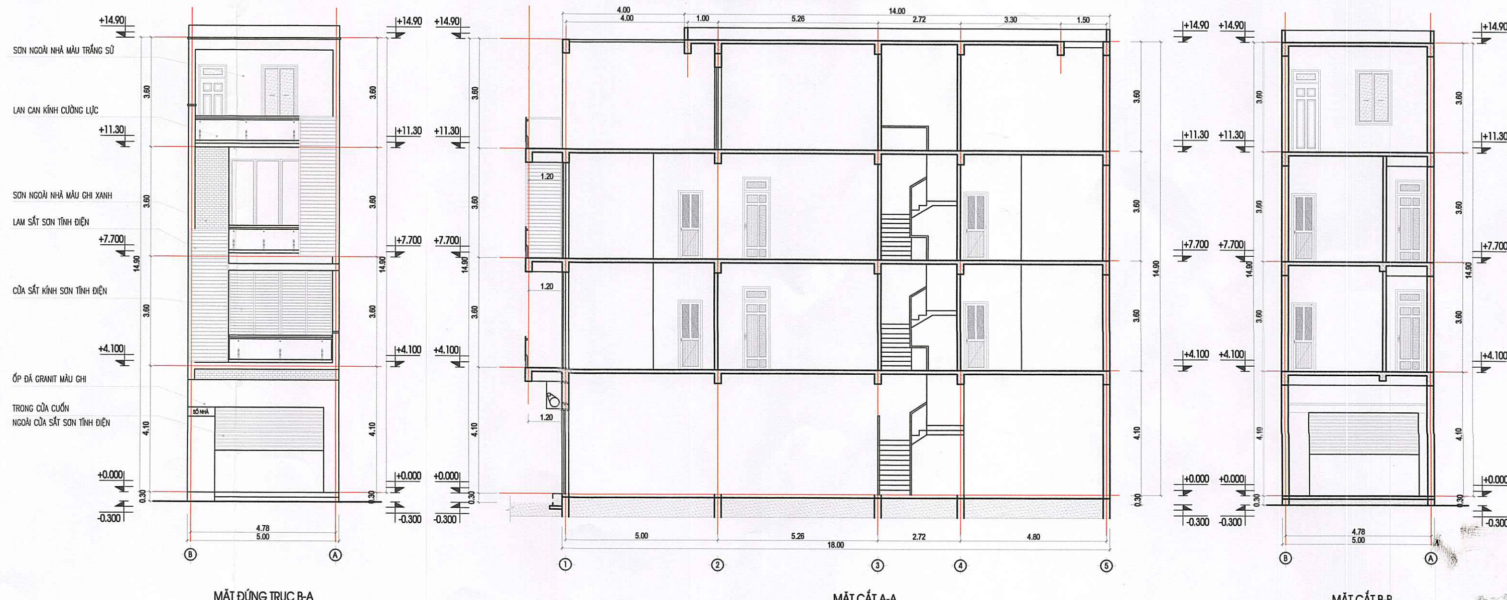
MẶT ĐƯNG TRỰC B-A
