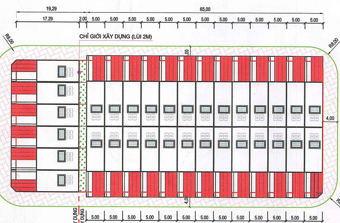
MẪU NHÀ ĐIỂN HÌNH
