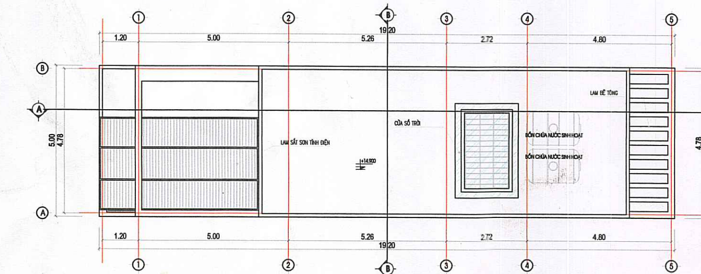
MẶT BẰNG Mái
