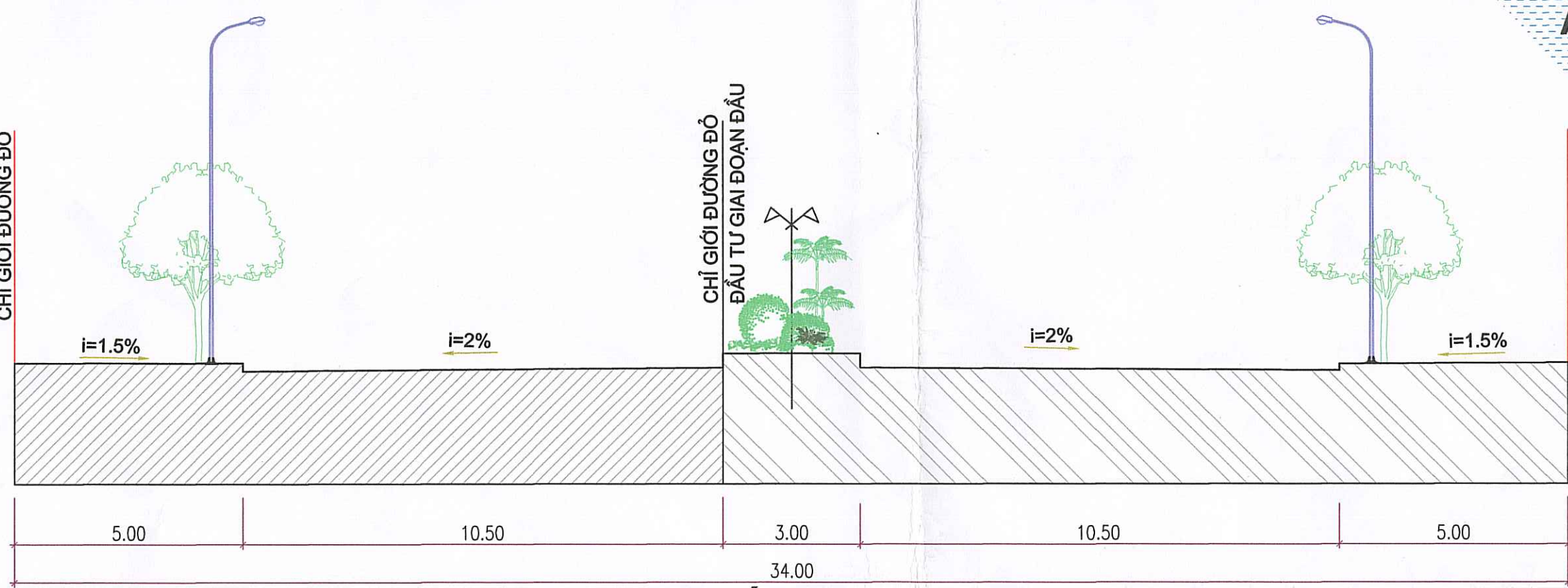
MẶT CẮT 1-1
