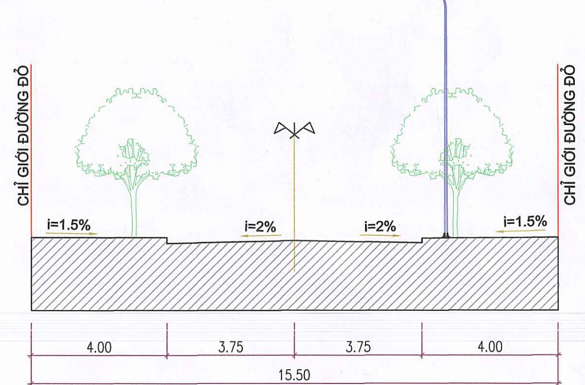
MẶT CẮT 2-2
