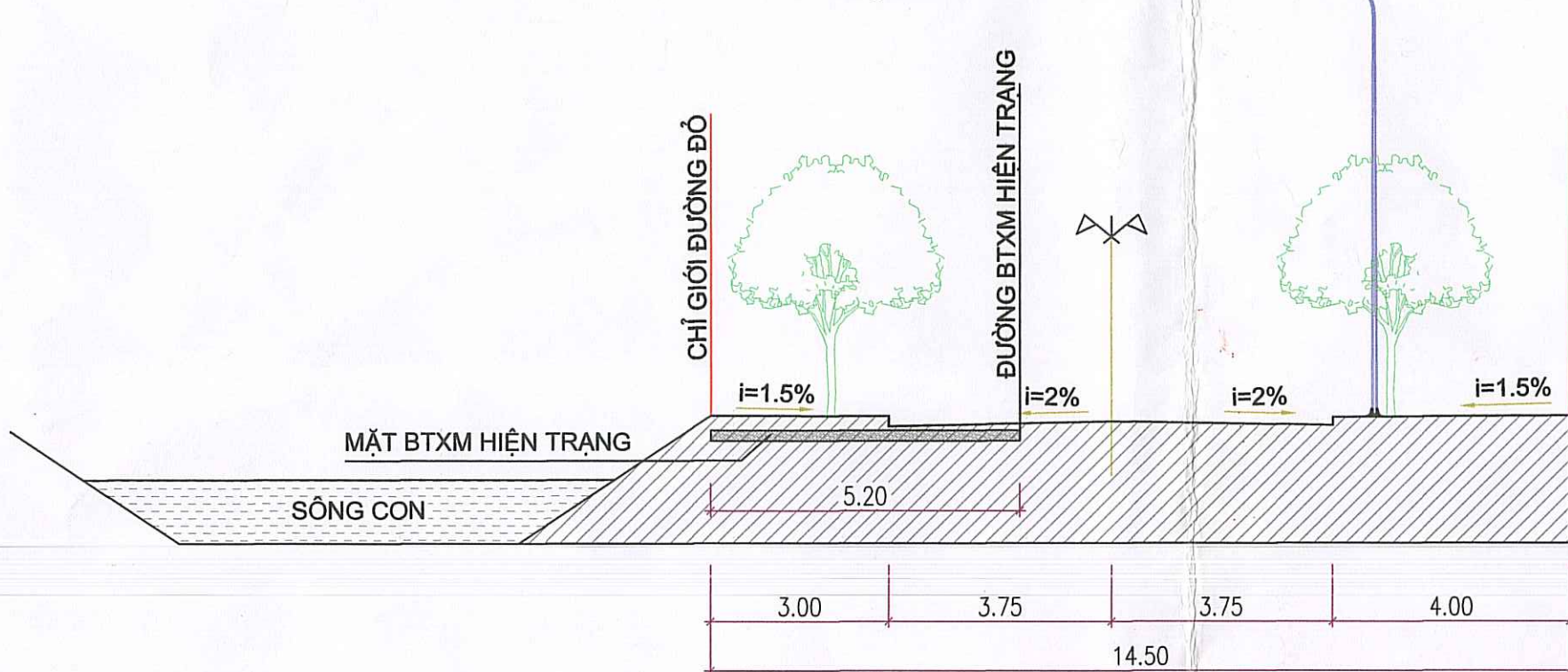
MẶT CẮT 3-3
