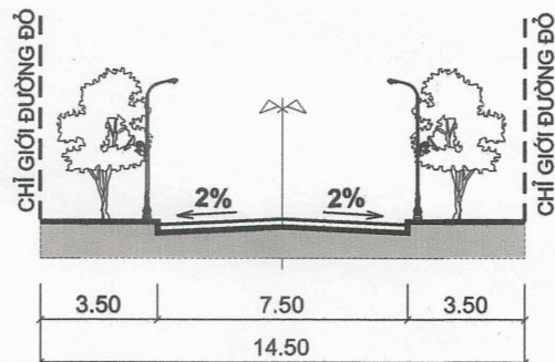
MẶT CẮT 1-1
