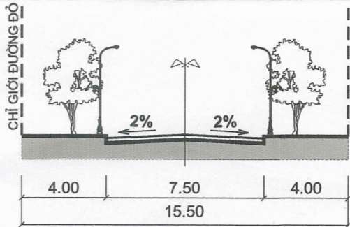
MẶT CẮT 2-2
