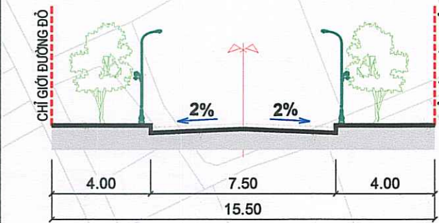
MẶT CẮT 1-1
